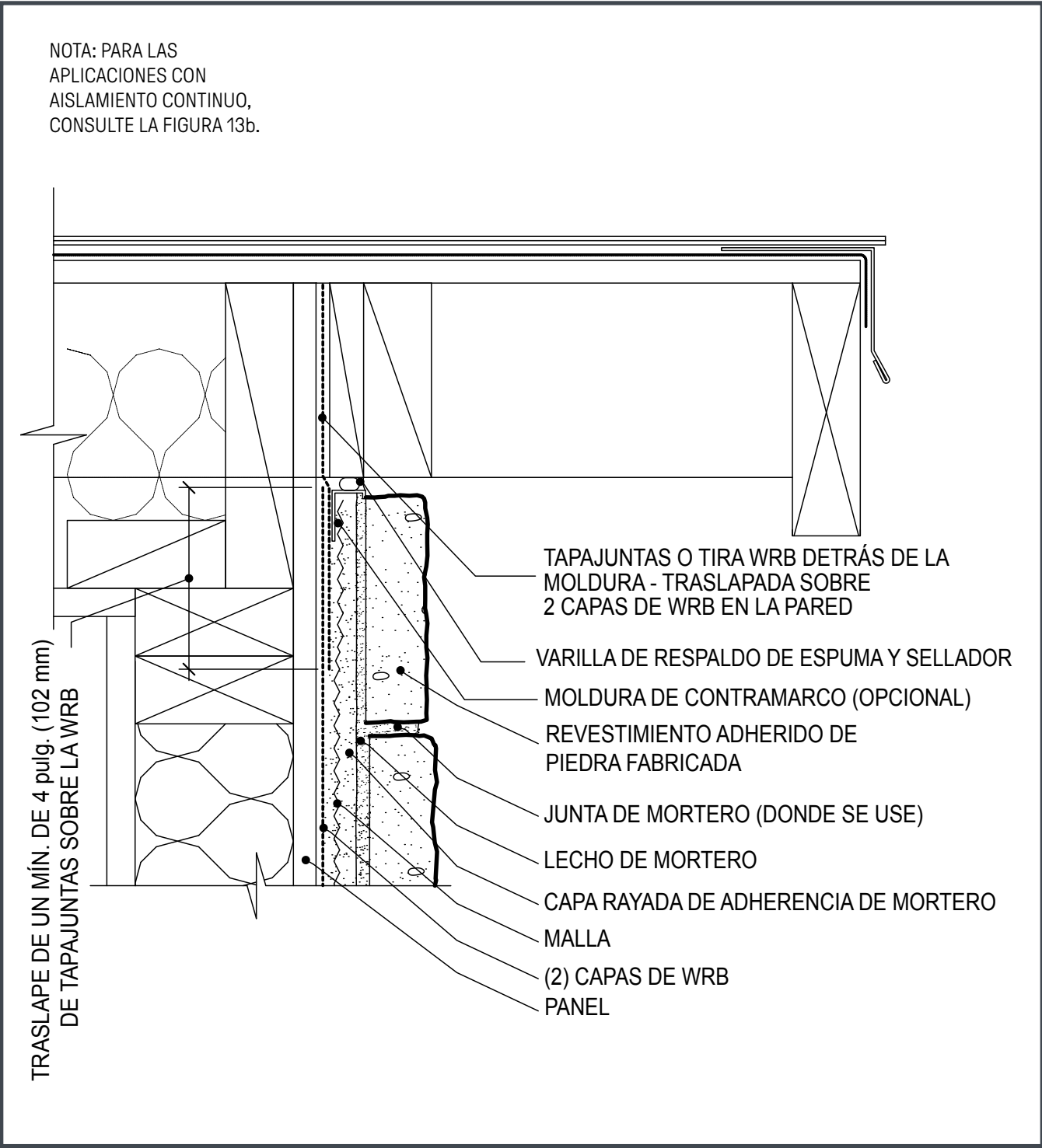
Figura 15. Remate lateral de techo - voladizo
