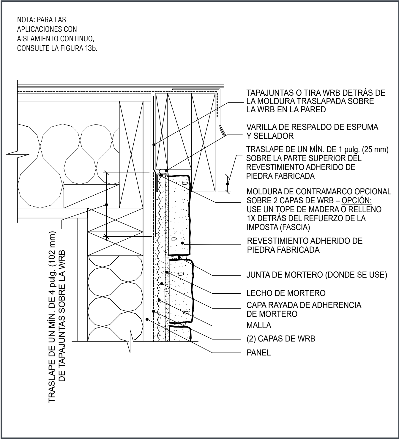
Figura 16. Remate lateral de techo - Al ras
