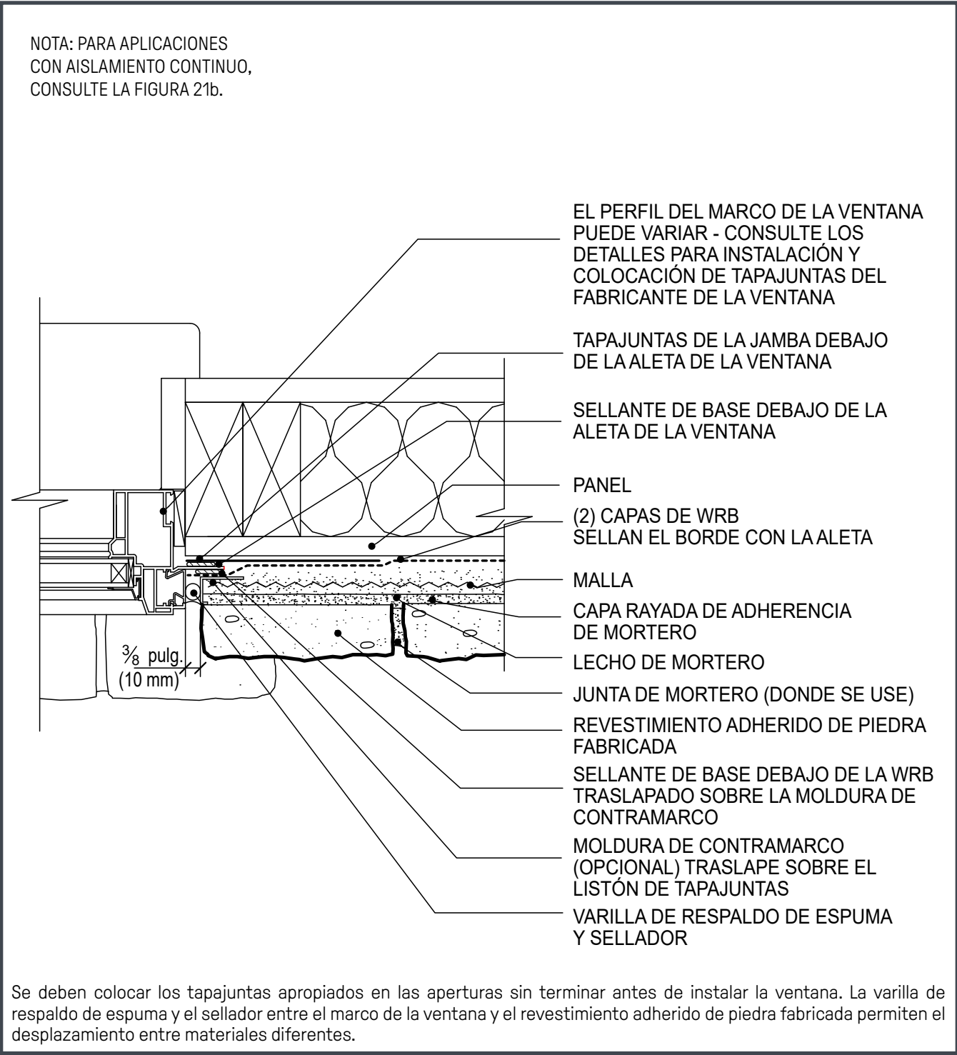
Figura 22. Jamba de la ventana
