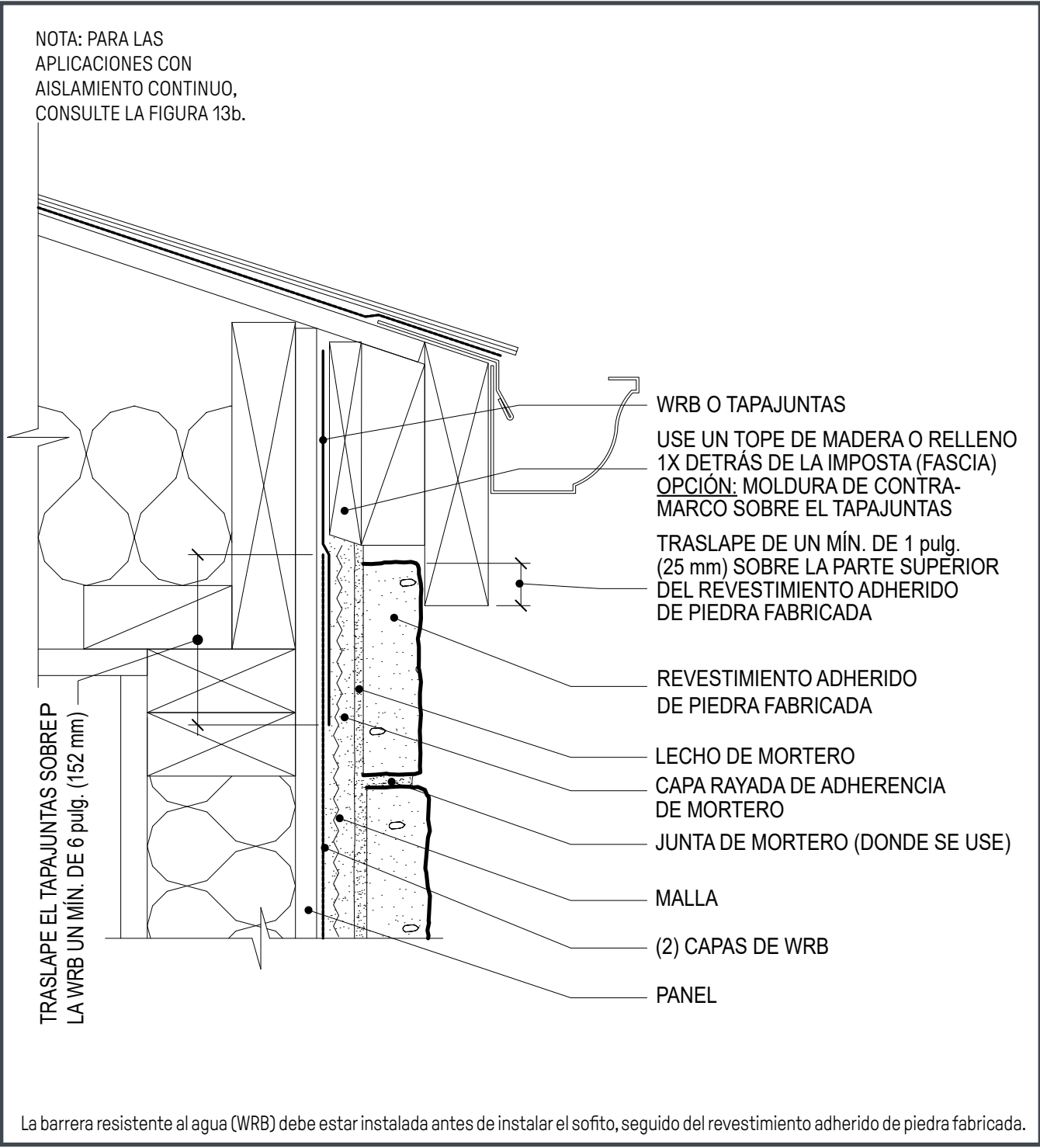
Figura 14. Alero abierto - Al ras
