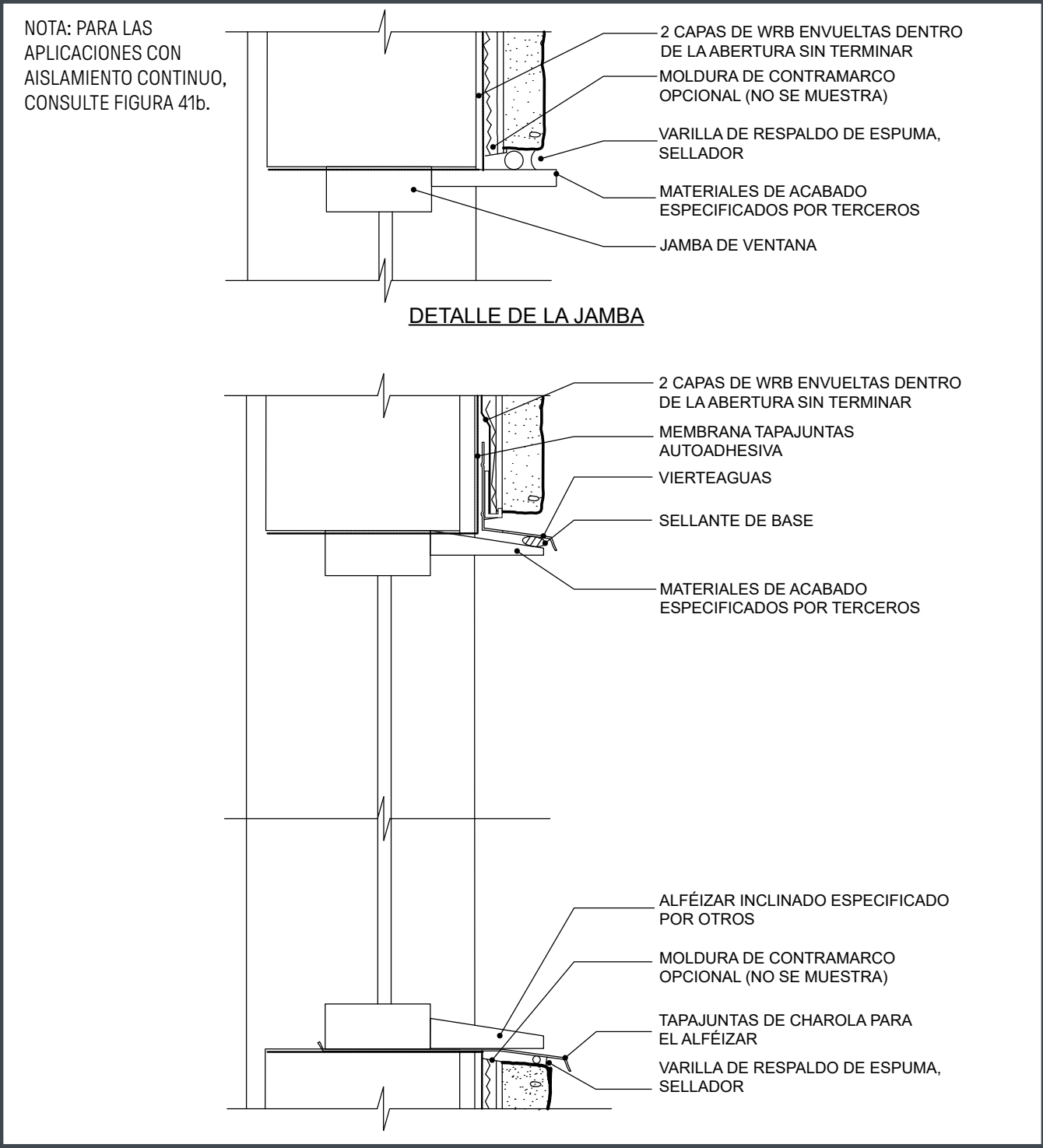
Figura 44. Ventana de escaparate comercial
