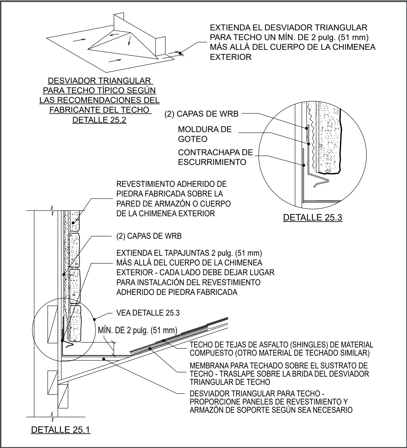
Figura 25. Desviador triangular para techo
