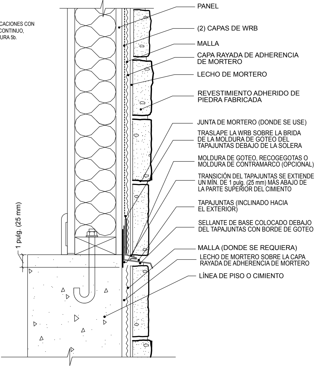
Figura 7. Muro de cimentación-Transición del AMSV cuando continúa hacia abajo hasta la cimentación
