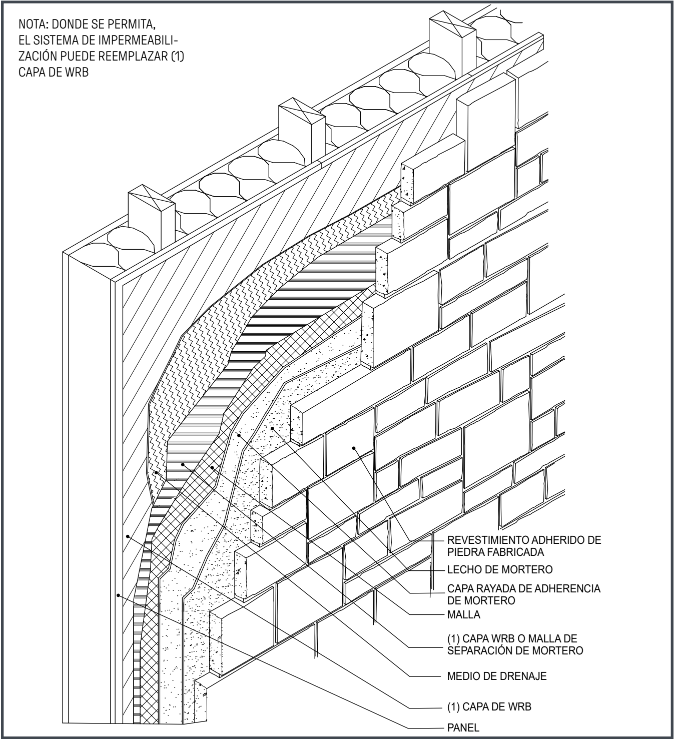
Figura 35. Muro con sistema de impermeabilización - Sistema de membrana
