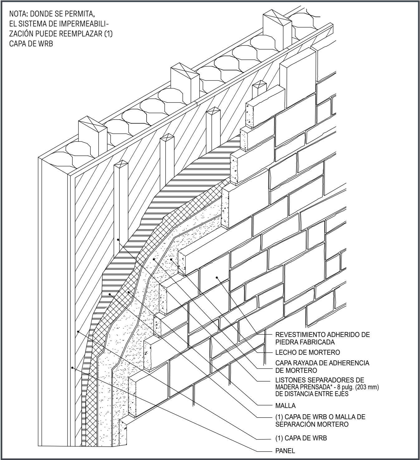
Figura 36. Muro con sistema de impermeabilización - Con listones
